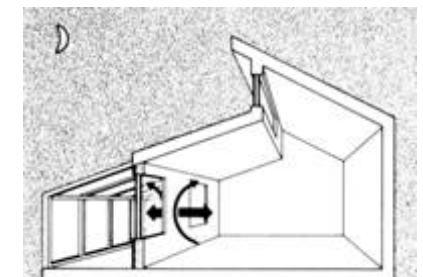
Espacio adosado de noche
