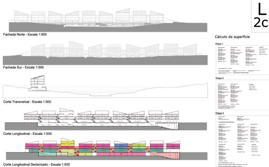
Fachada Gral. y Cortes
