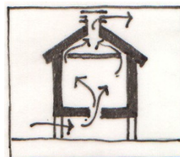
Chimenea solar
