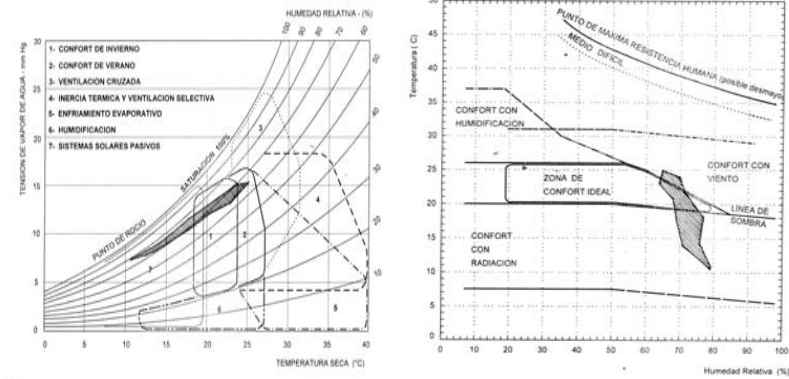
Diagramas Bioclimáticos de Givini y Ogyay
