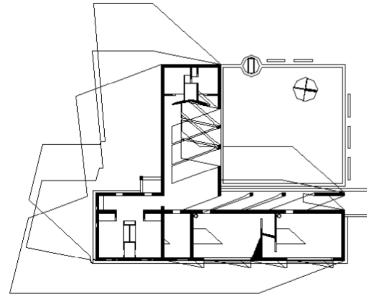
Asoleamiento 21 de Junio:10, 12,14 Hs
