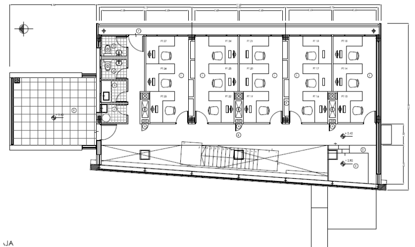
Planta alta
