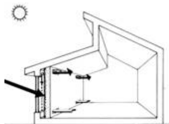
Muro Tromba de día
