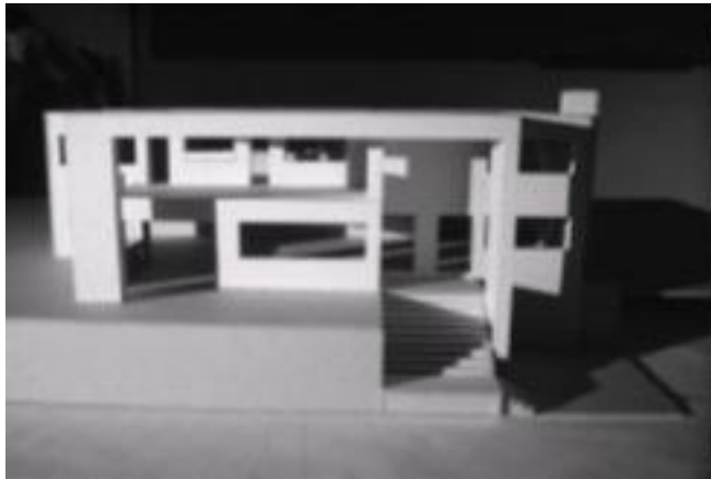
Heliódón 21 de Junio: 10 Hs
