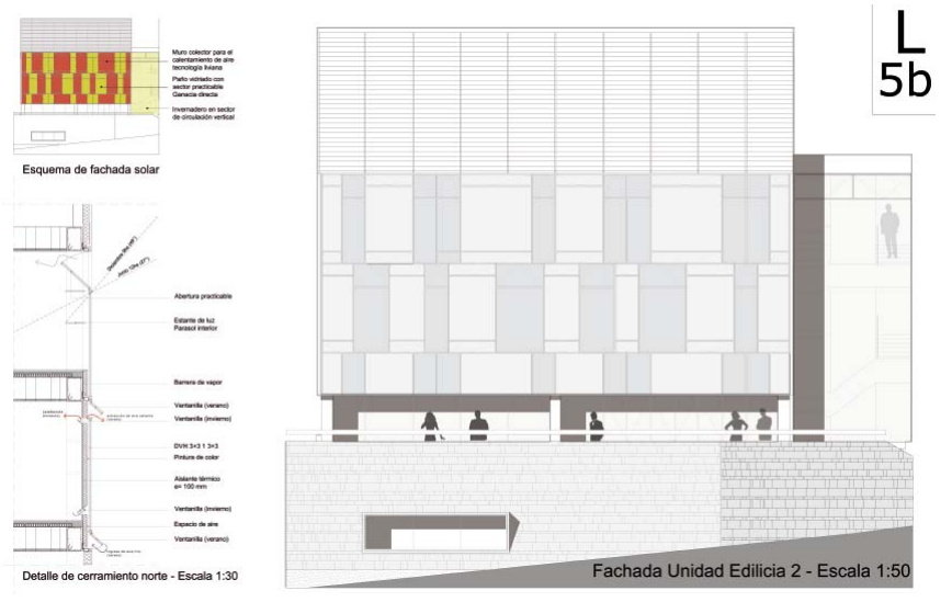
Esquema fachada y Corte
