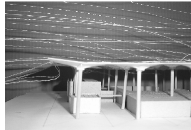
Análisis de ventilación en el túnel de vientos.
