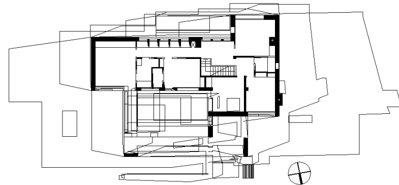
Asoleamiento 21 de Diciembre 08,10,12,14,16 Hs
