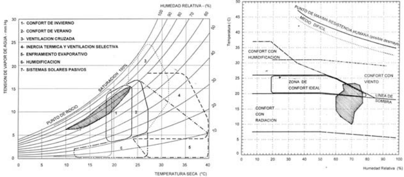
Diagramas Bioclimáticos de Givini y Ogyay
