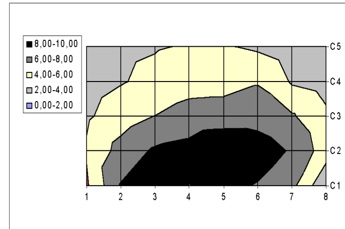
Estudio de iluminación natural en el cielo artificial
