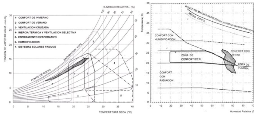
Diagramas Bioclimáticos de Givini y Ogyay
