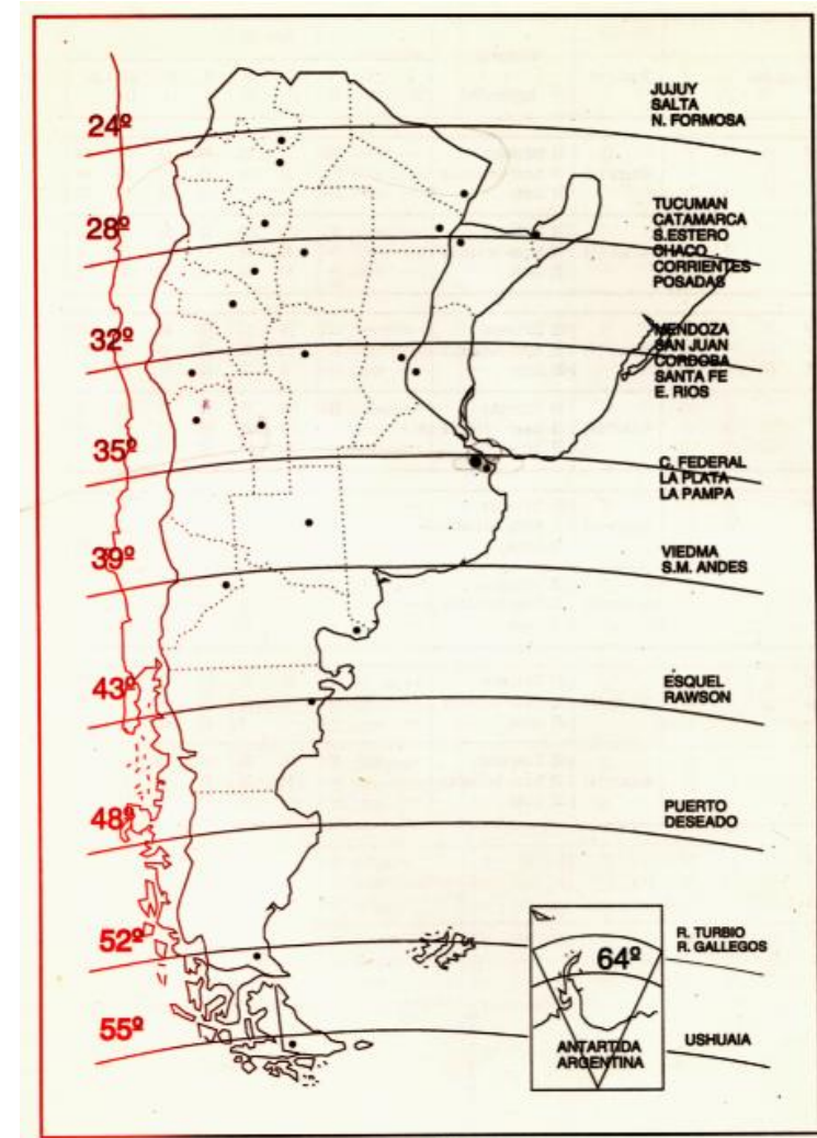
Latitudes seleccionadas para la determinación de Altura y Acimut solar
