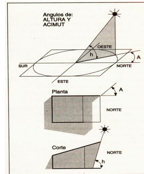
Altura y Acimut
